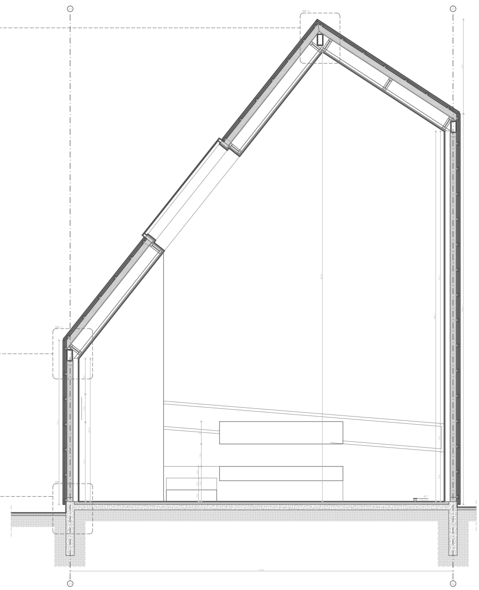
ESCANTILLON A1
